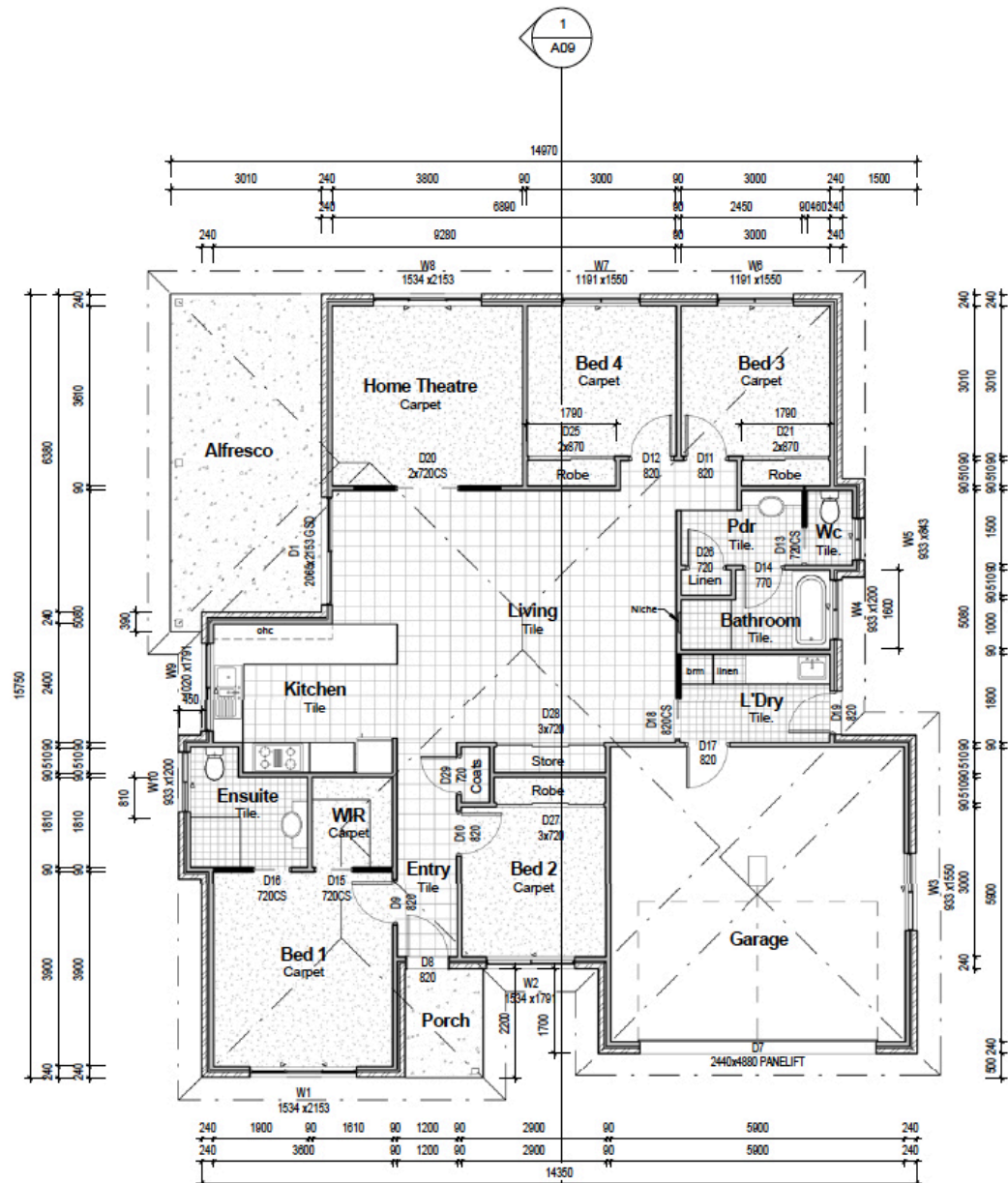
1 Floor Plan 1 : 100
